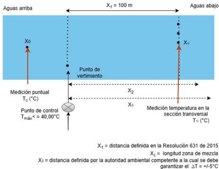
FIGURA 14. DETERMINACIÓN DE \Delta T_{100} Y X_3
